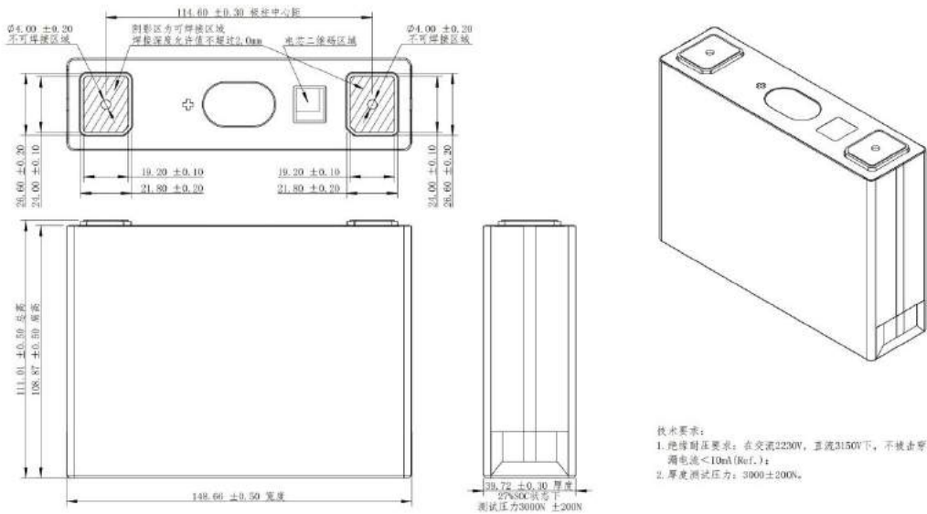
Figure 7 电池尺寸 /mm
