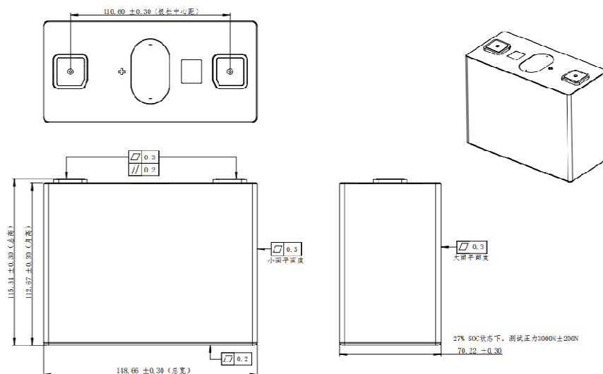
Figure 7 电池尺寸 /mm
