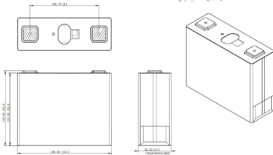
图 7 电池尺寸/mm
