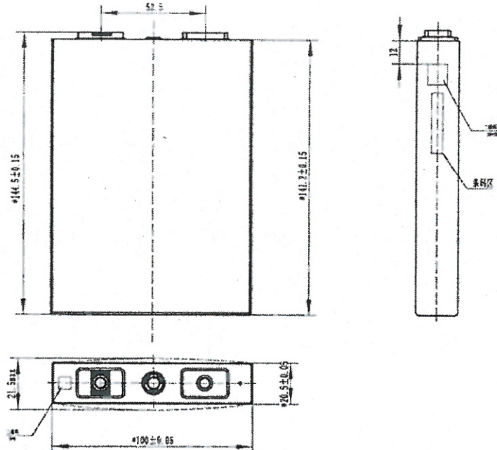
图 A.1 电池尺寸图
